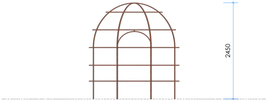
2 Elevation
