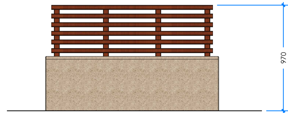
2 ELEVATION Scale: 1:20
