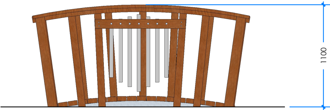
2 ELEVATION Scale: 1:25
