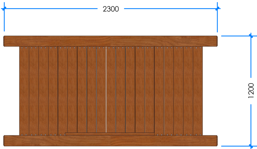
3 TOP Scale: 1:25
