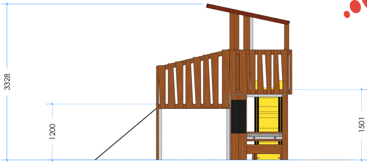
2 Elevation
