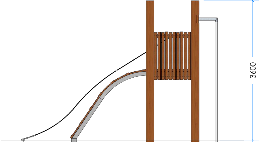
2 Elevation
