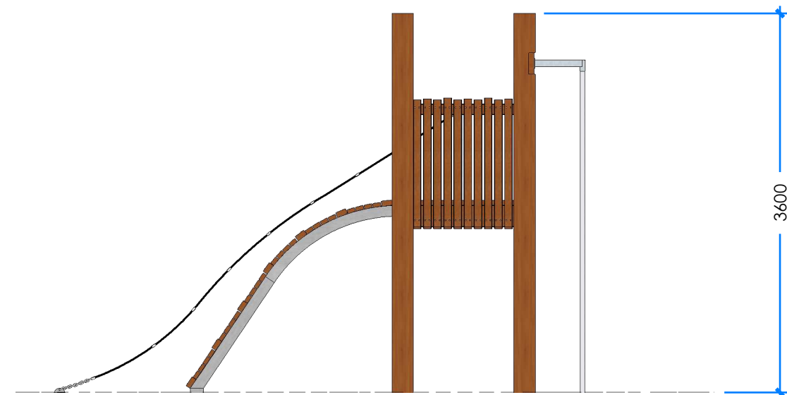
2 ELEVATION Scale: 1:50
