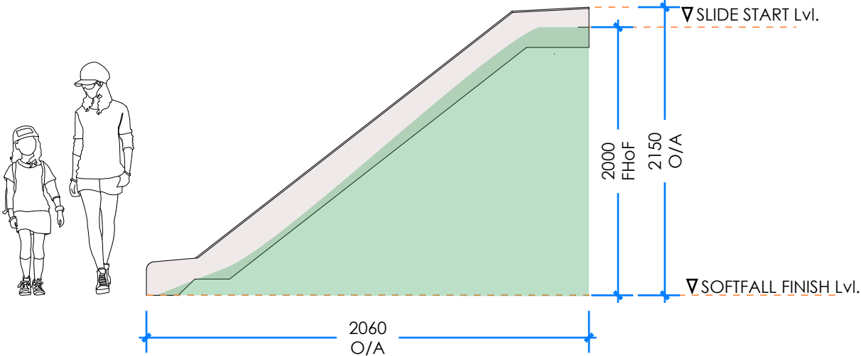
2 ELEVATION LEFT Scale: 1:40
