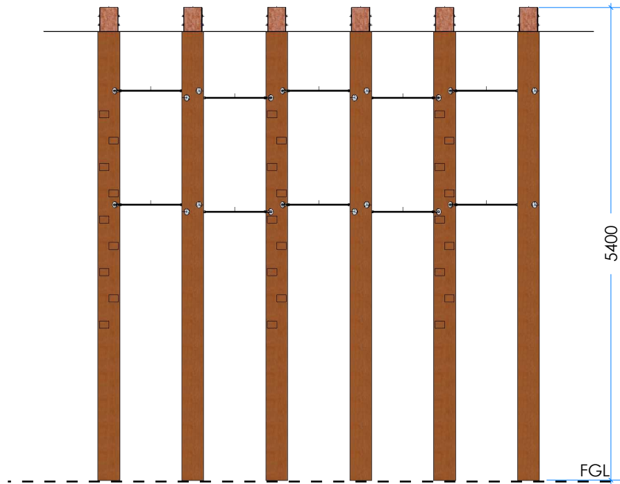
2 Elevation
