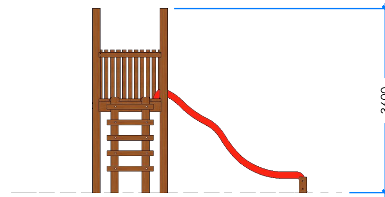
2 ELEVATION Scale: 1:75
