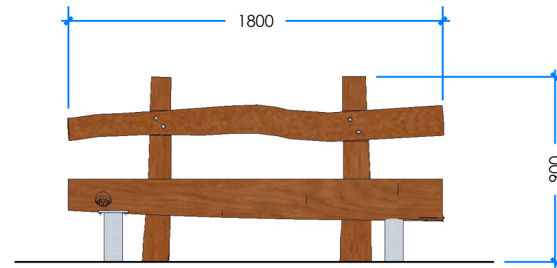
2 ELEVATION Scale: 1:25
