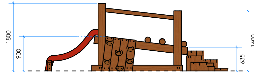
2 ELEVATION Scale: 1:50
