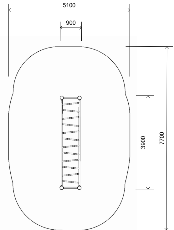
3 Top View Scale: 1:100
