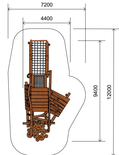
3 Top View Scale: 1:200
