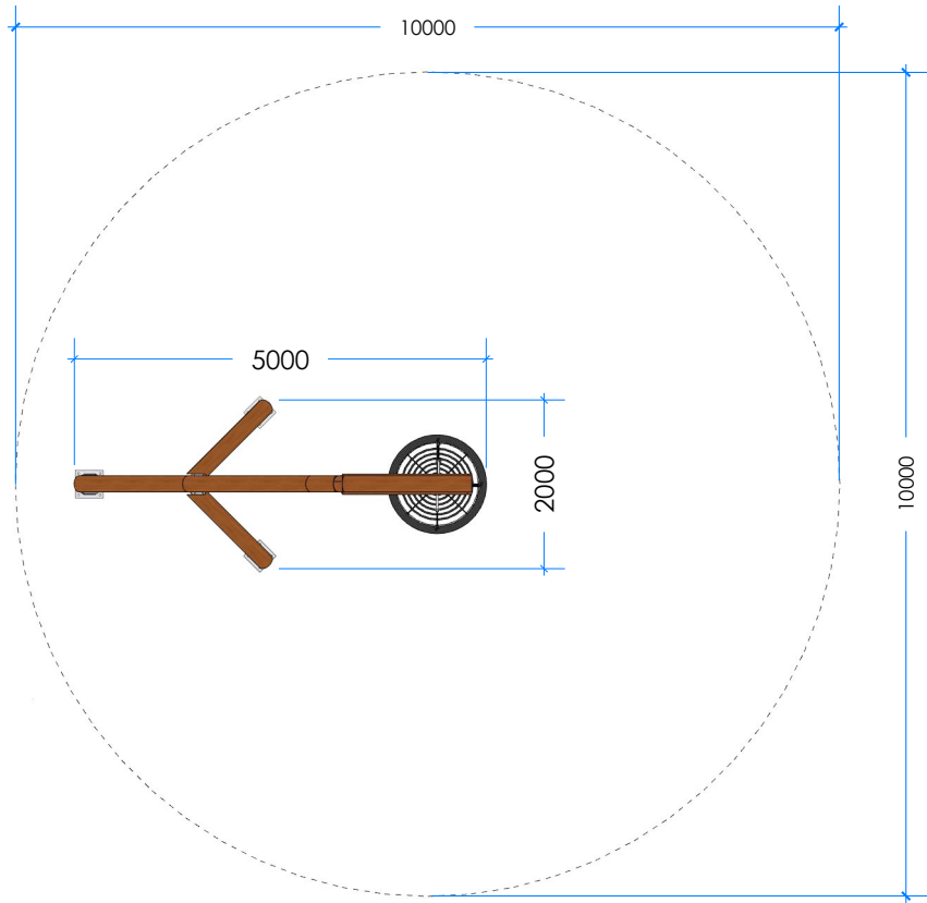
3 TOP 1:100
