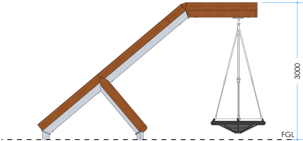
2 ELEVATION 1:50
