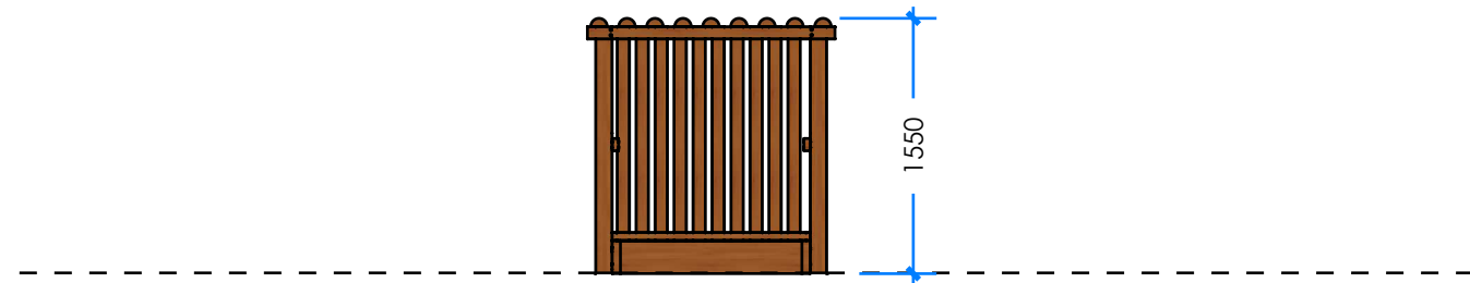
2 ELEVATION Scale: 1:50
