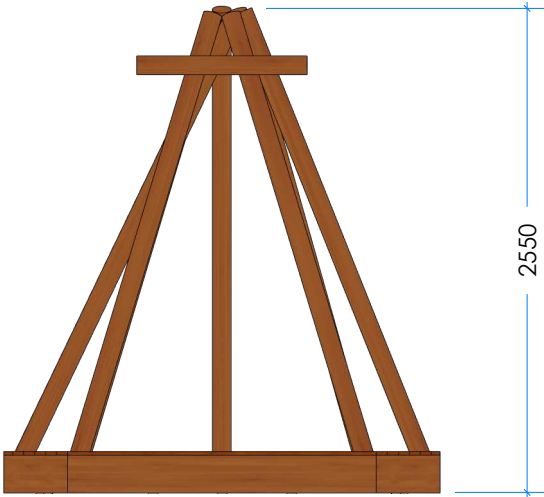
2 Elevation
