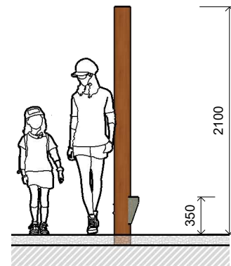
2 Front View Scale: 1:50
