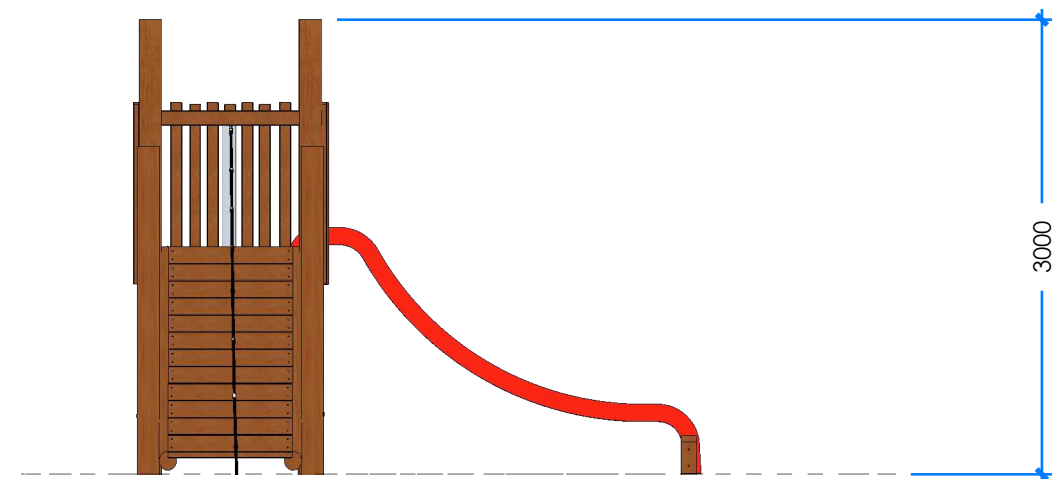
2 ELEVATION Scale: 1:50
