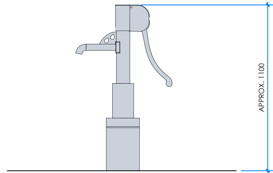
2 ELEVATION Scale: 1:50
