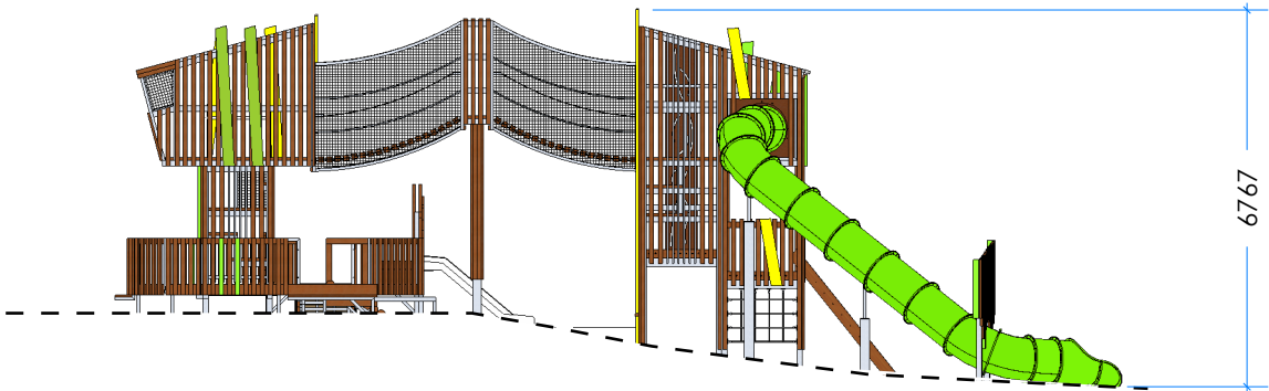
2 Elevation Scale: 1:150
