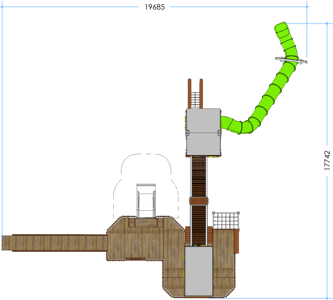
3 Top Scale: 1:150
