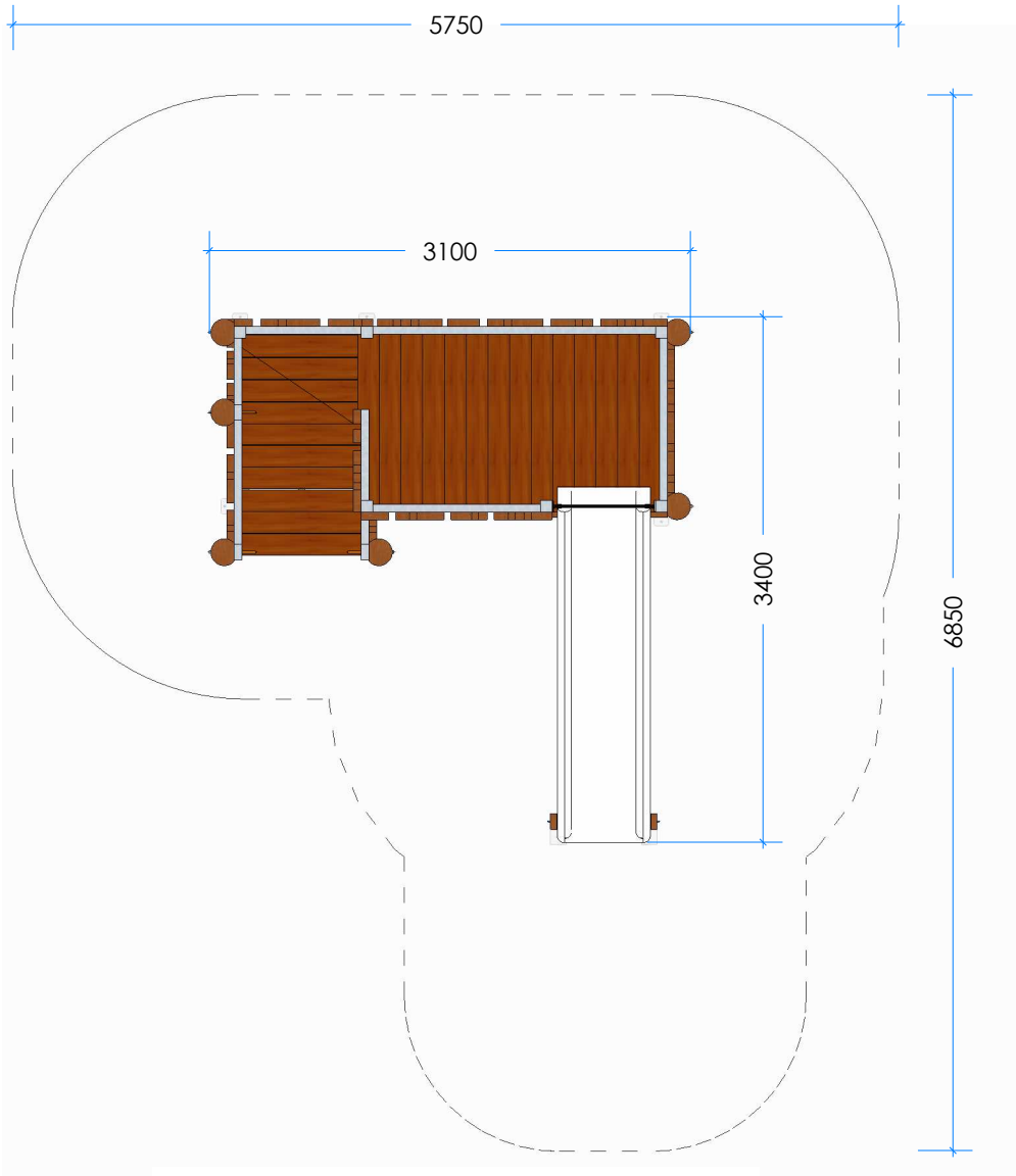
3 Top
