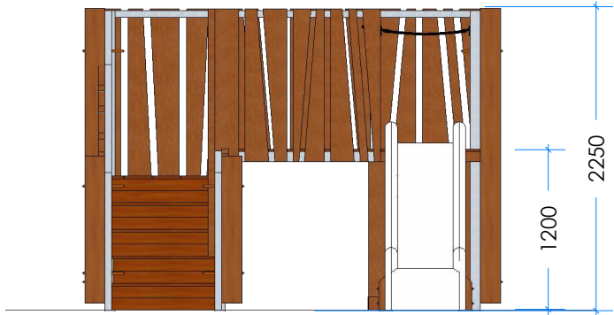
2 Elevation
