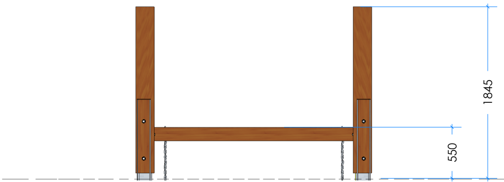
2 Elevation Scale: 1:40
