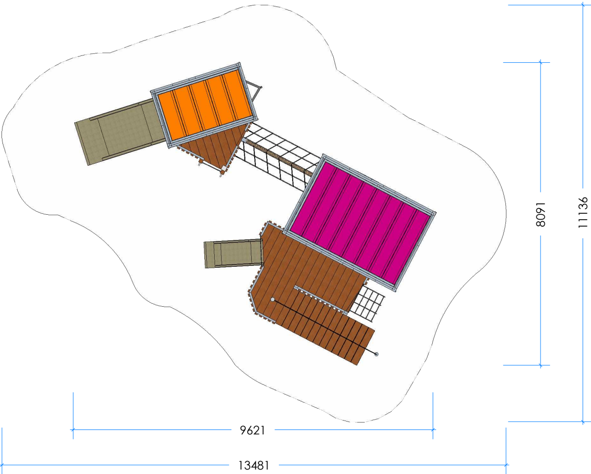
3 Top Scale: 1:100
