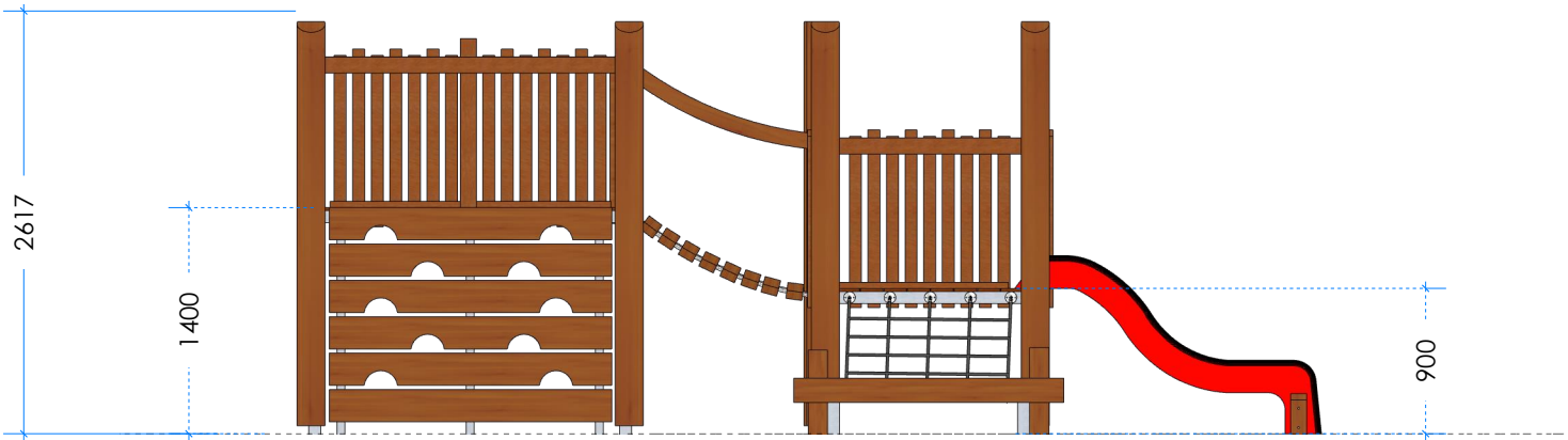
2 Elevation
