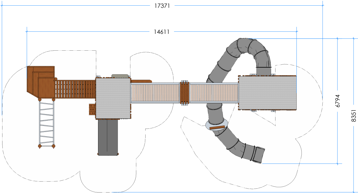
3 Top Scale: 1:100
