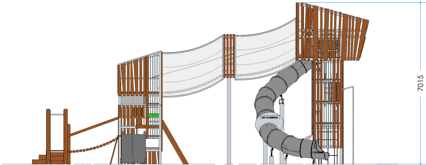
2 Elevation Scale: 1:100
