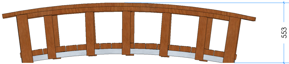
2 Elevation
