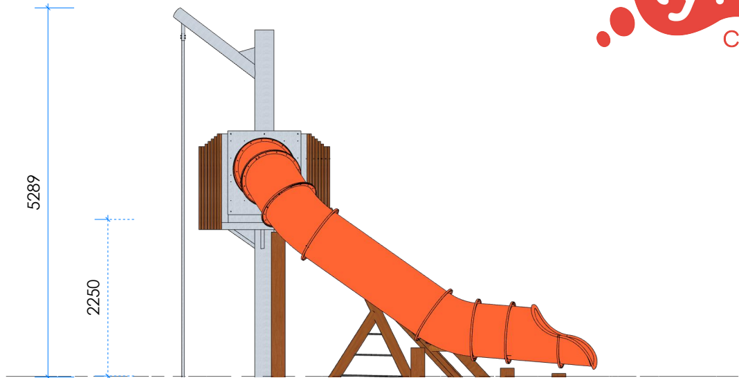
2 Elevation
