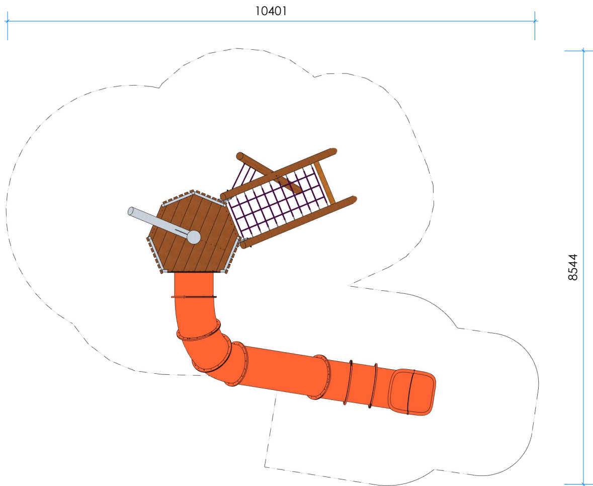
3 Top
