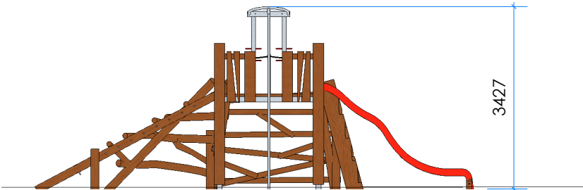
2 Elevation
