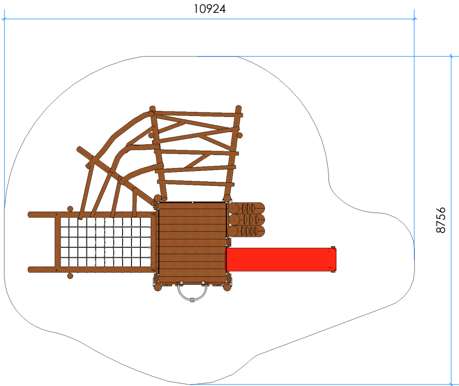
3 Top
