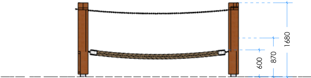
2 Elevation
