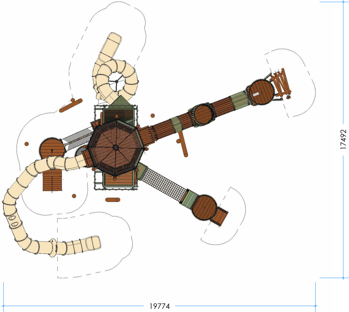
3 Top Scale 1:150
