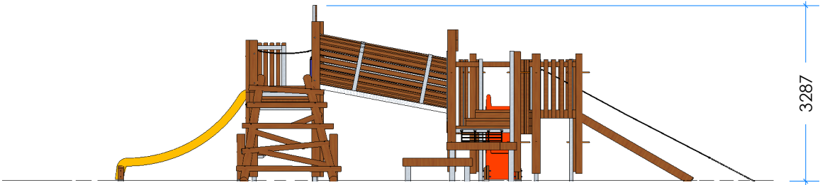
2 Elevation Scale: 1:100
