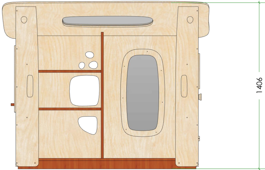
2 Elevation
