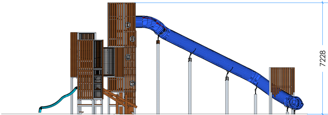
2 Elevation Scale: 1:150
