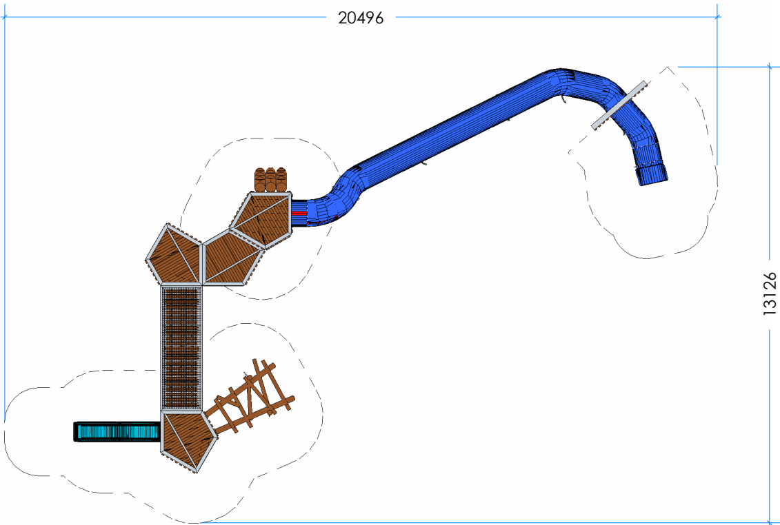
3 Top Scale: 1:150
