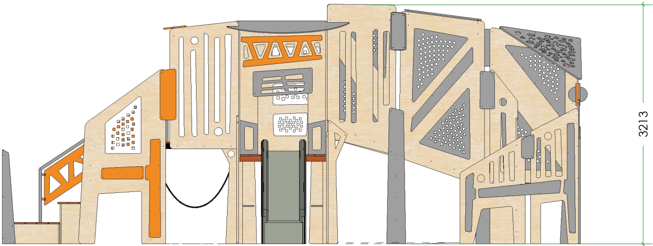
2 Elevation
