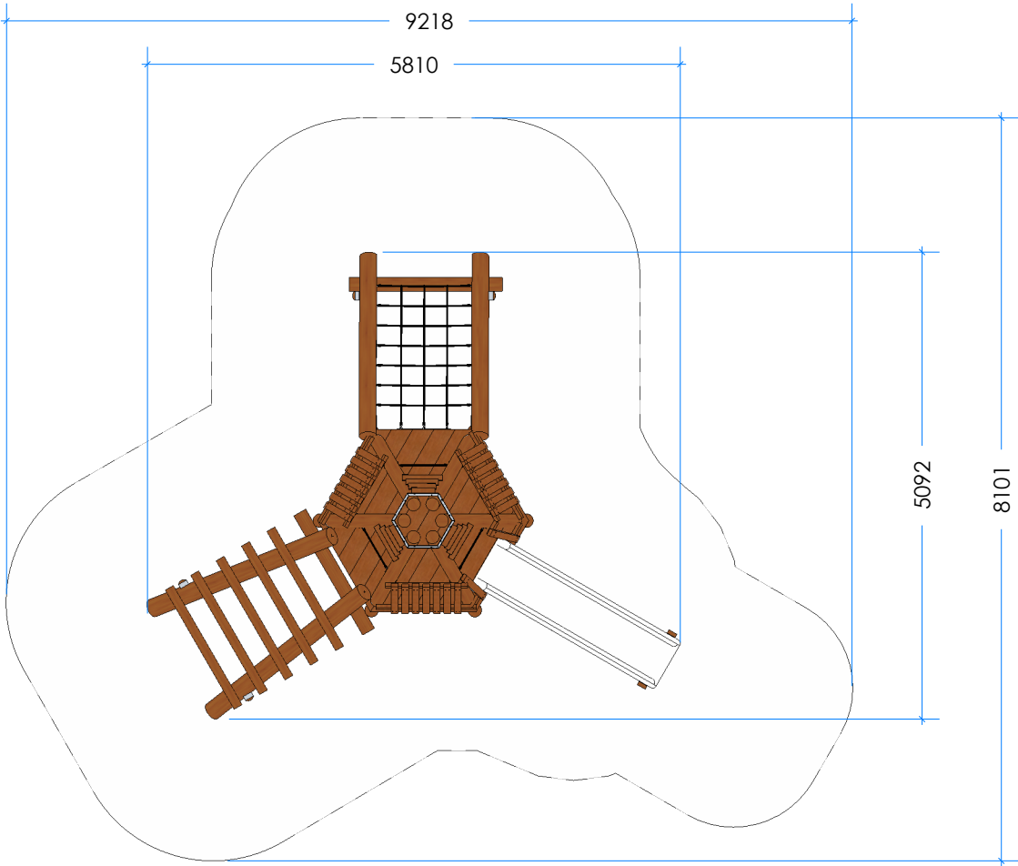
3 Top Scale: 1:75
