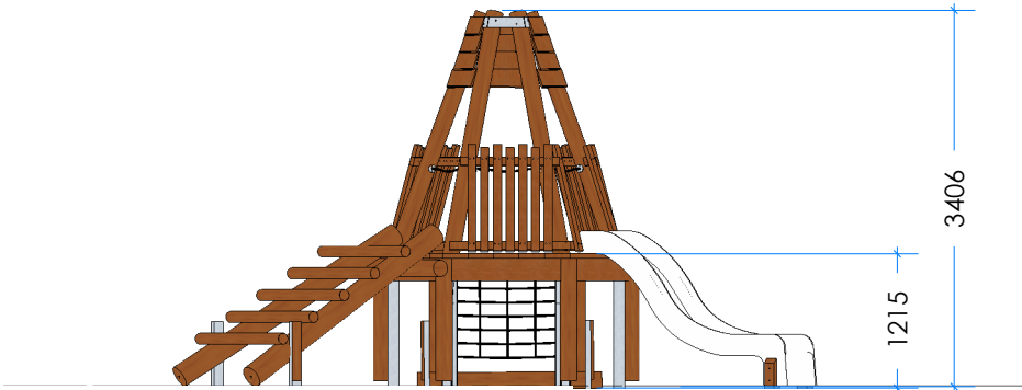
2 Elevation Scale: 1:75
