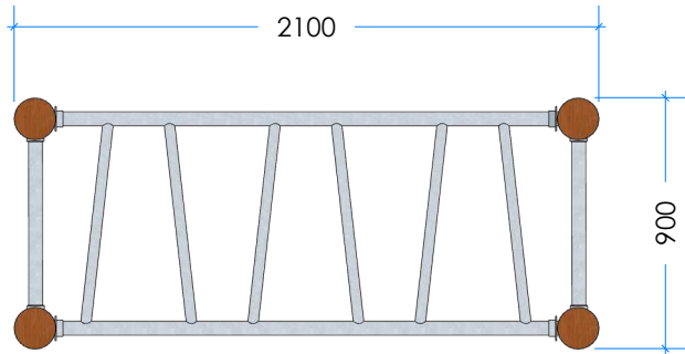
3 Top
