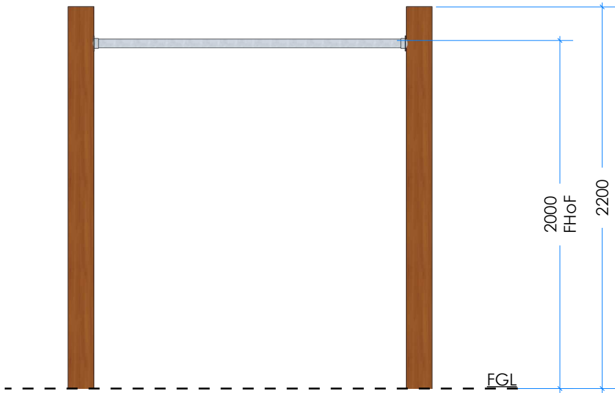
2 Elevation
