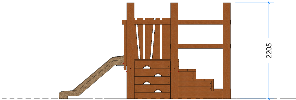
2 Elevation Scale: 1:50
