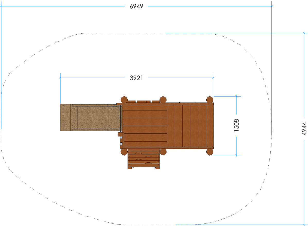
3 Top Scale: 1:50
