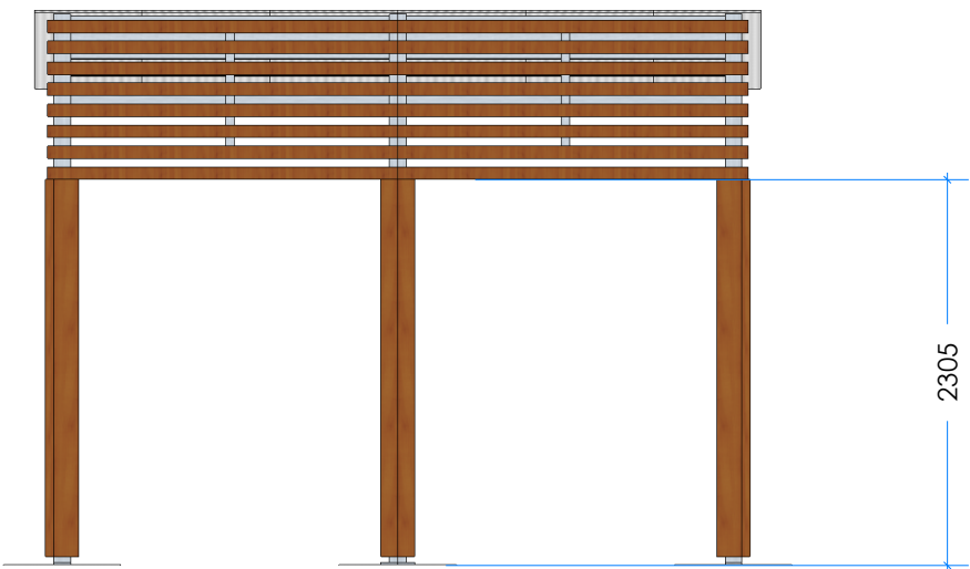
2 ELEVATION Scale: 1:50
