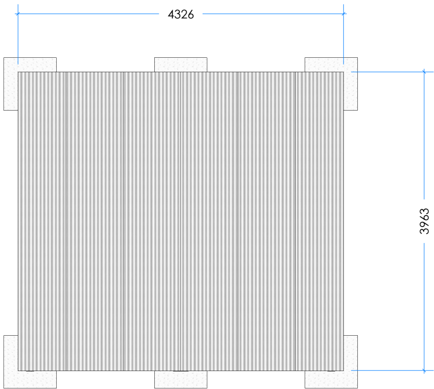
3 TOP Scale: 1:50
