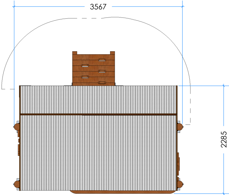
3 Top Scale: 1:50
