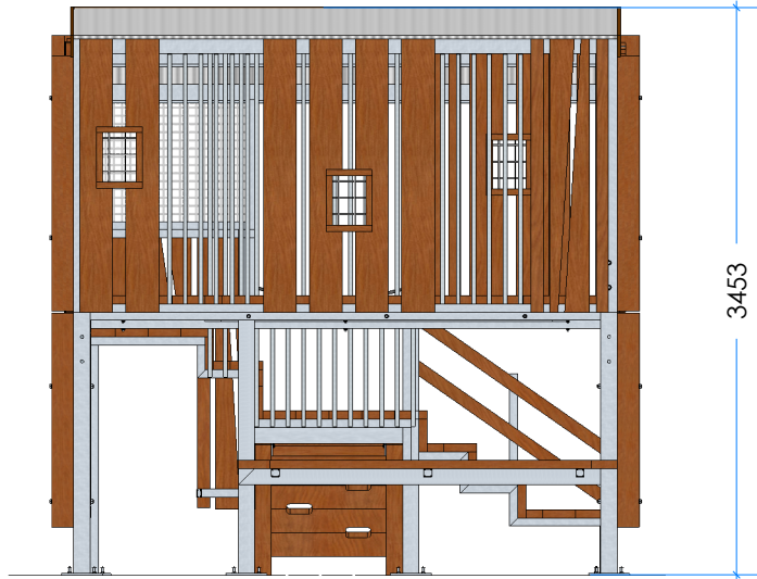
2 Elevation Scale: 1:50
