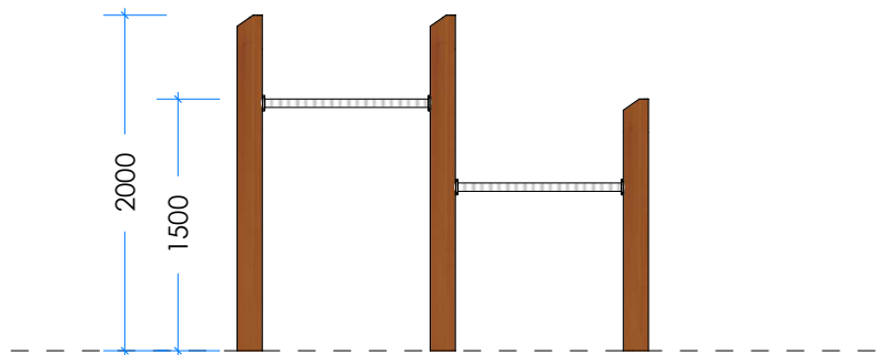
2 Elevation
