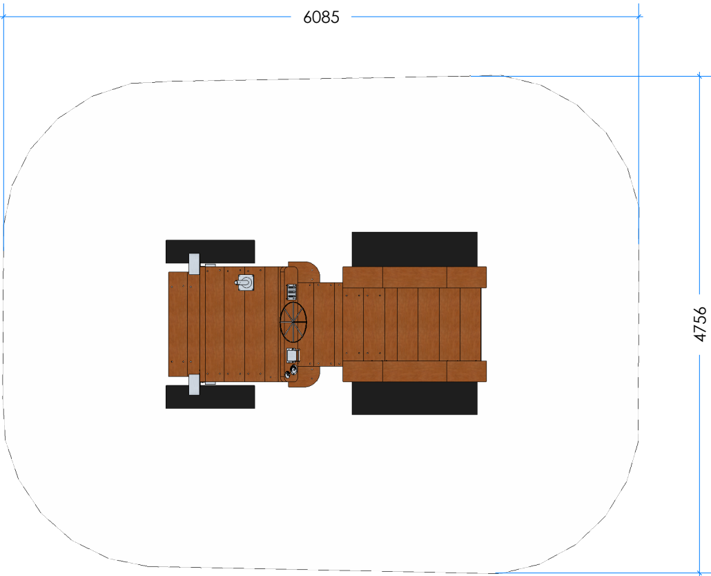
3 Top Scale: 1:50
