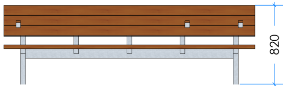
2 Elevation Scale: 1:40
