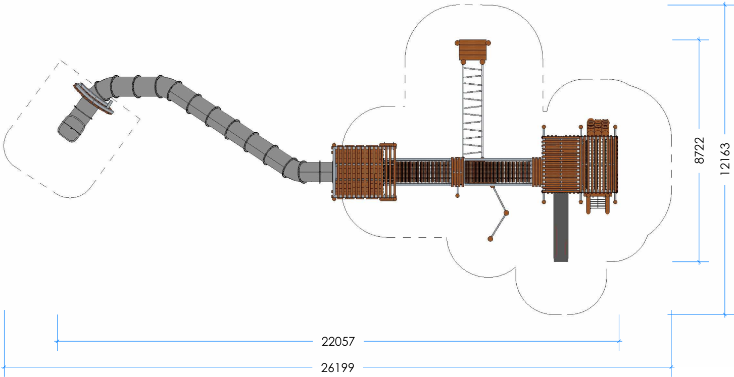
3 Top Scale 1:150
