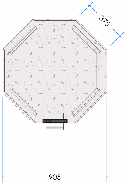
3 Top Scale: 1:20
