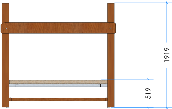
2 Elevation Scale: 1:50
