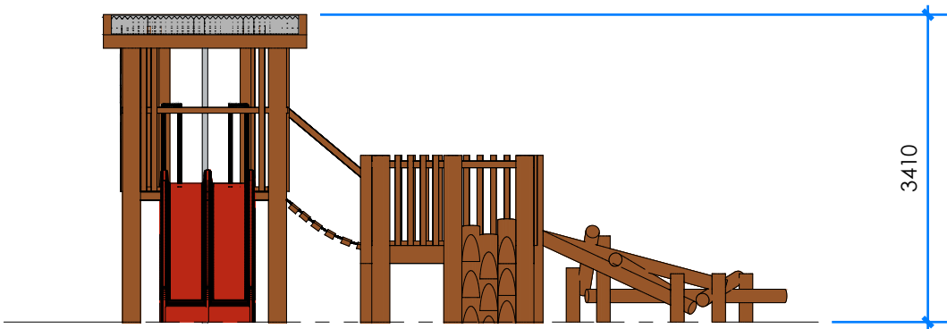
2 ELEVATION Scale: 1:75
