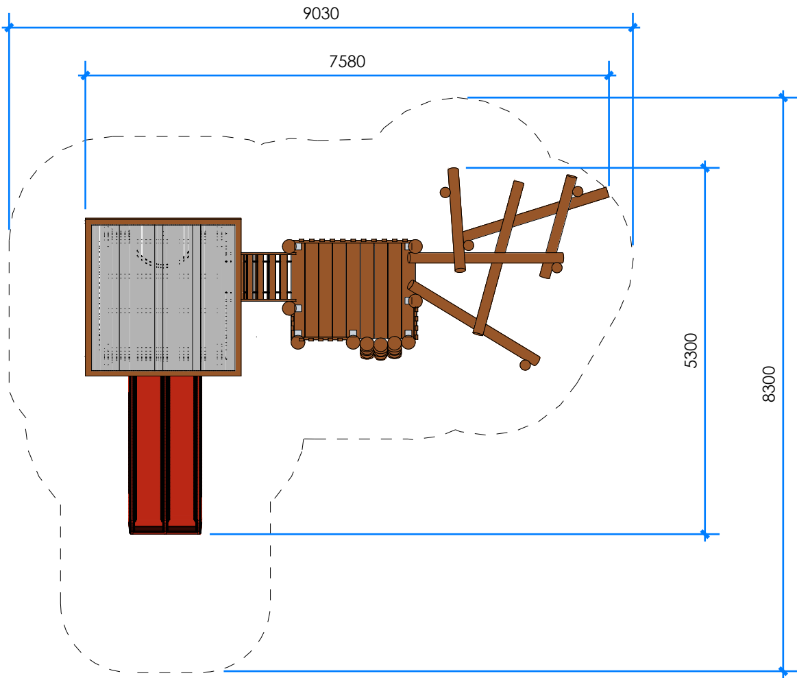
3 TOP Scale: 1:75
