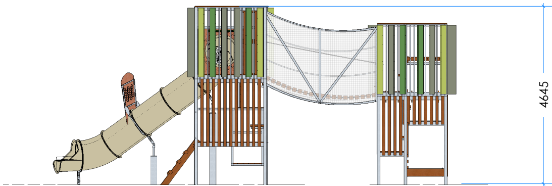
2 Elevation Scale: 1:100
