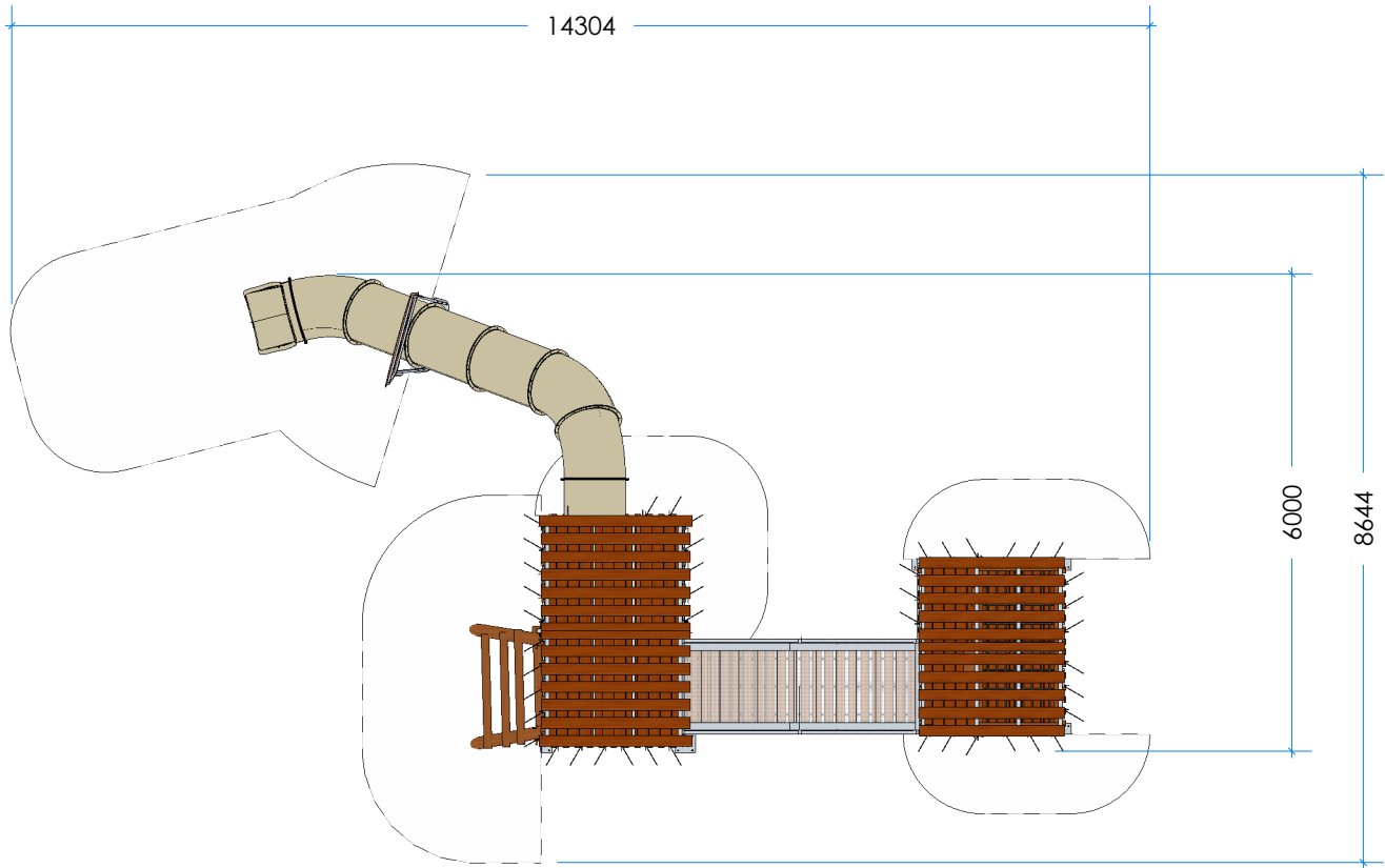
3 Top Scale: 1:100
