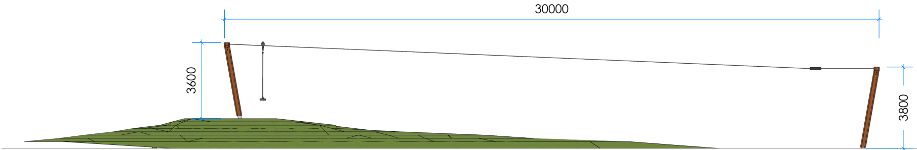
2 Elevation
