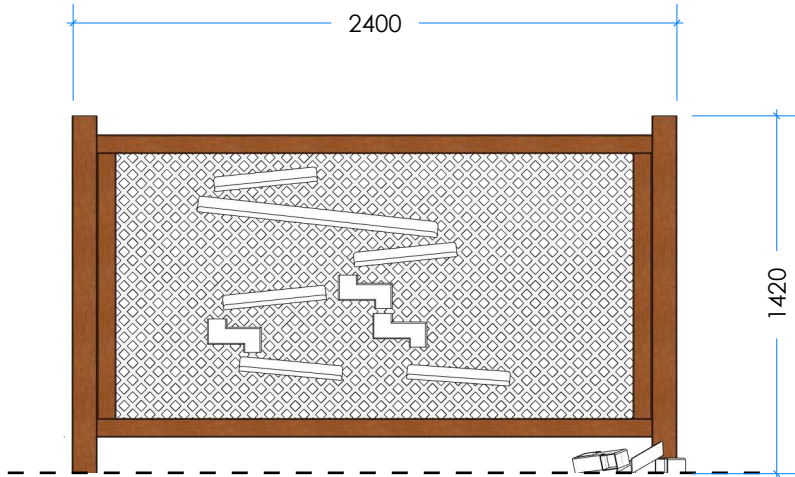
2 Elevation
