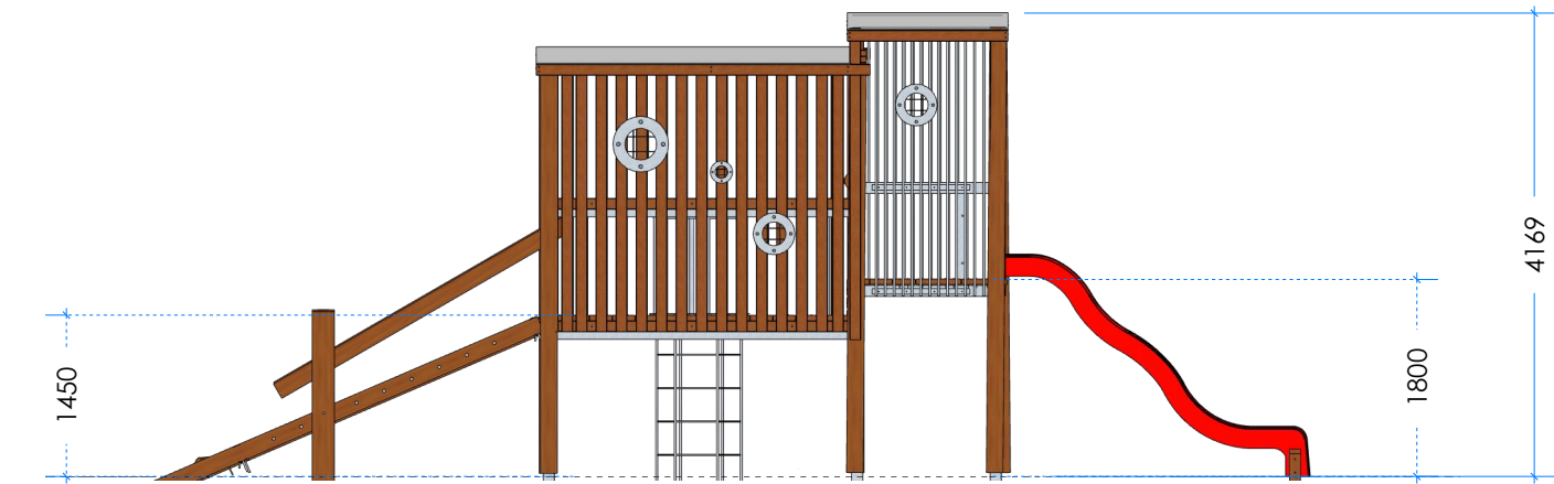
2 Elevation
