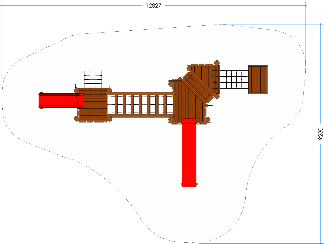
3 Top Scale: 1:75
