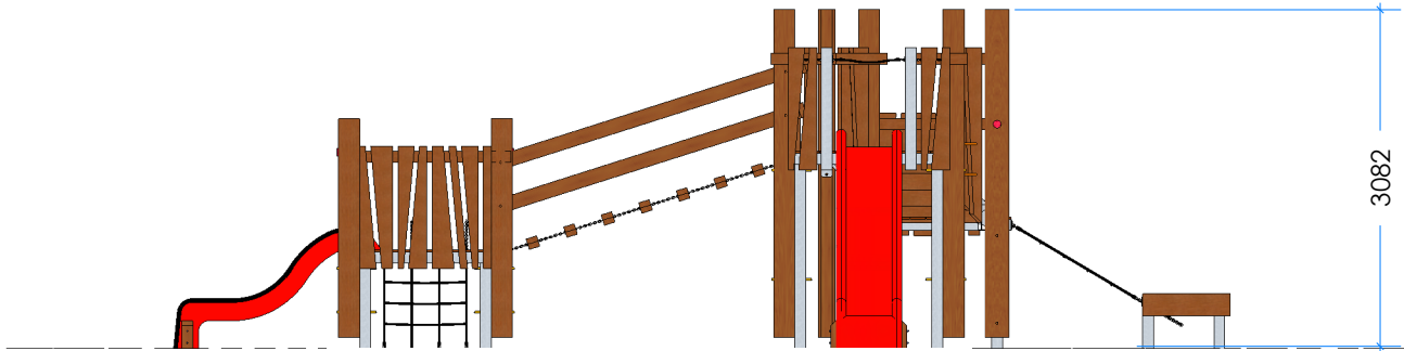
2 Elevation Scale: 1:75
